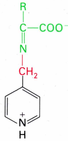
Ketimine
